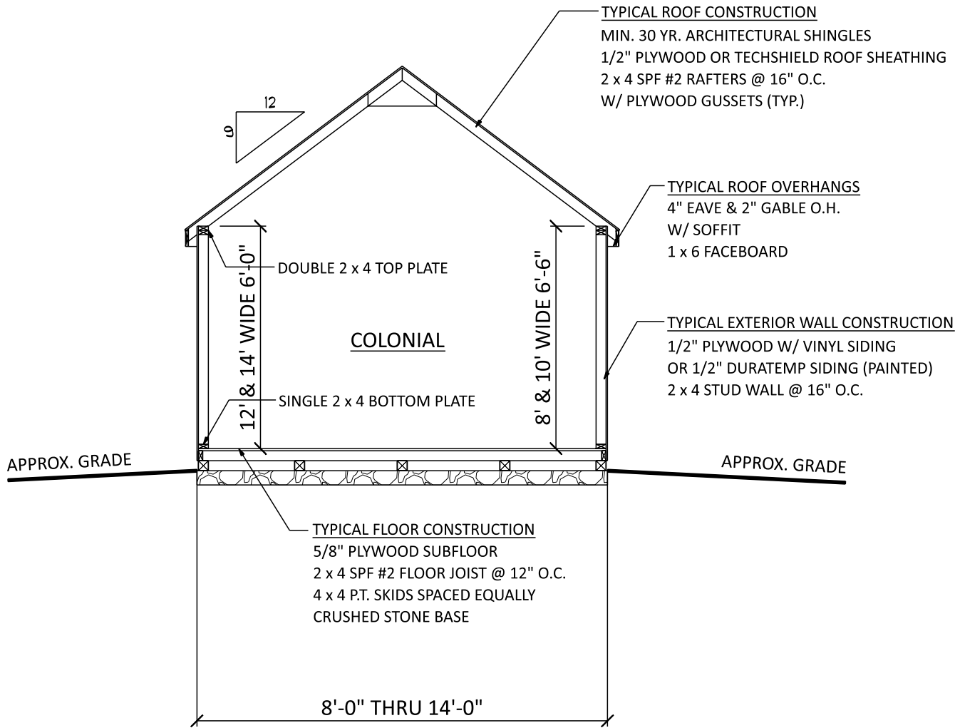
Section SCALE: 1/4" = 1'-0"
